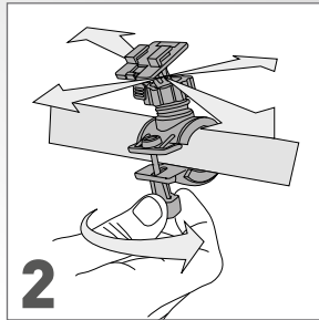
2 Avvitare al tubolare del manubrio e regolare a piacere l'inclinazione della basetta
